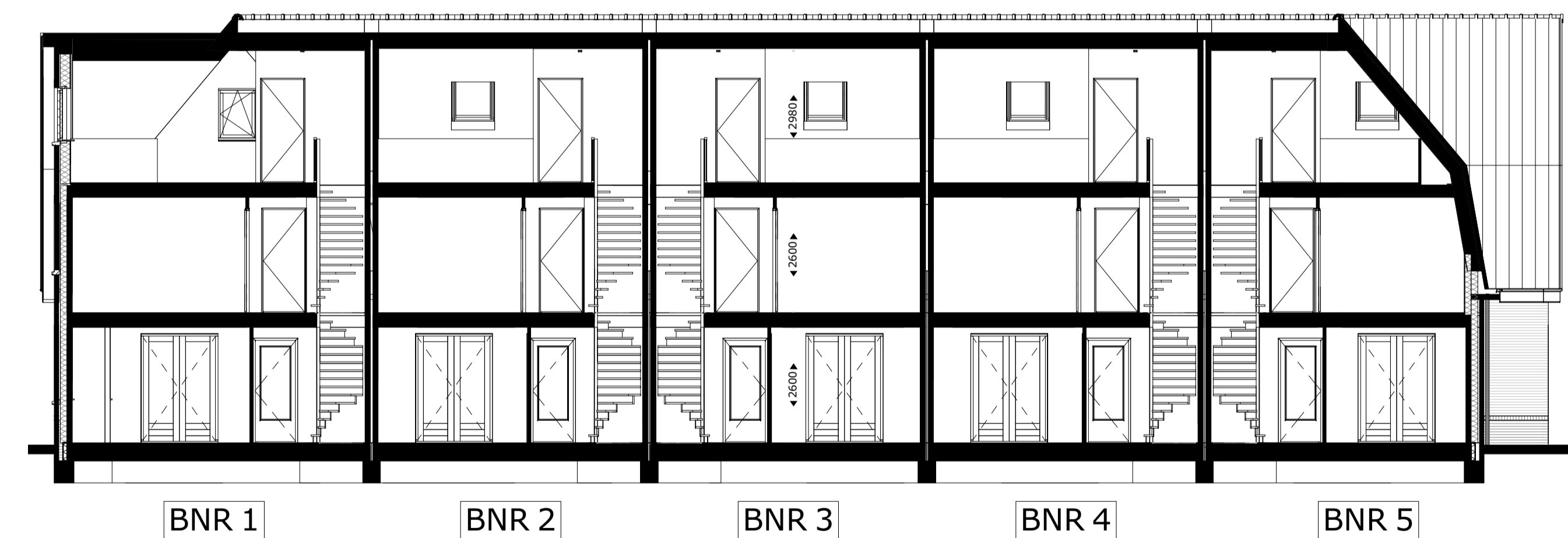
doorsnede A
