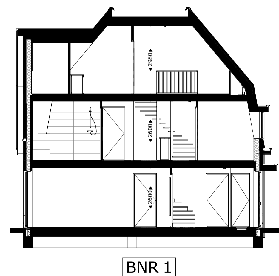
doorsnede B
