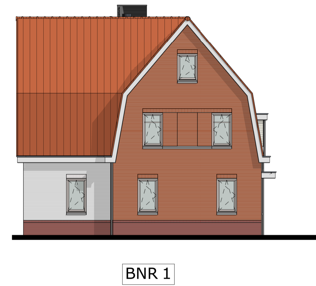
linker zijgevel
