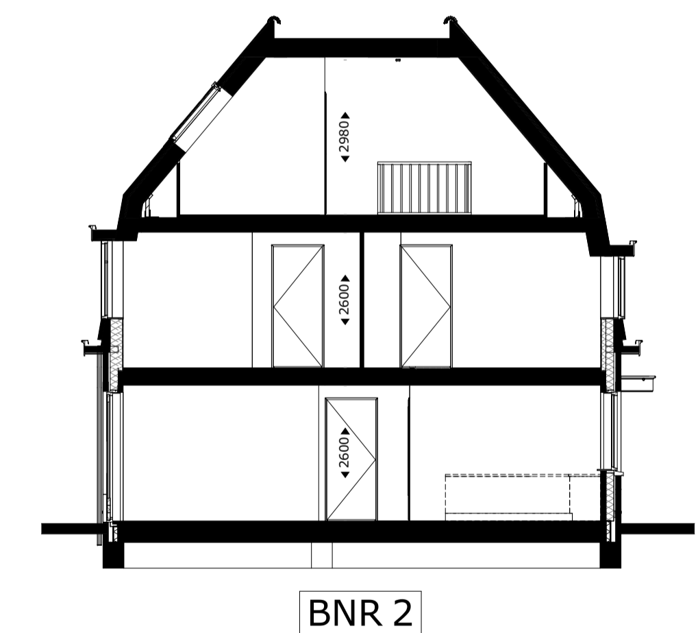
doorsnede C
