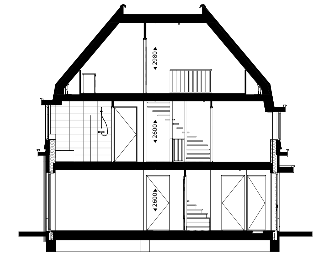
doorsnede D
